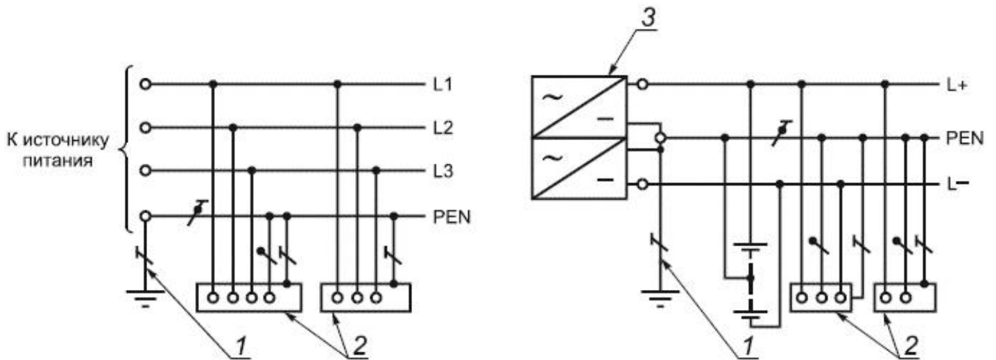
а) переменного тока
