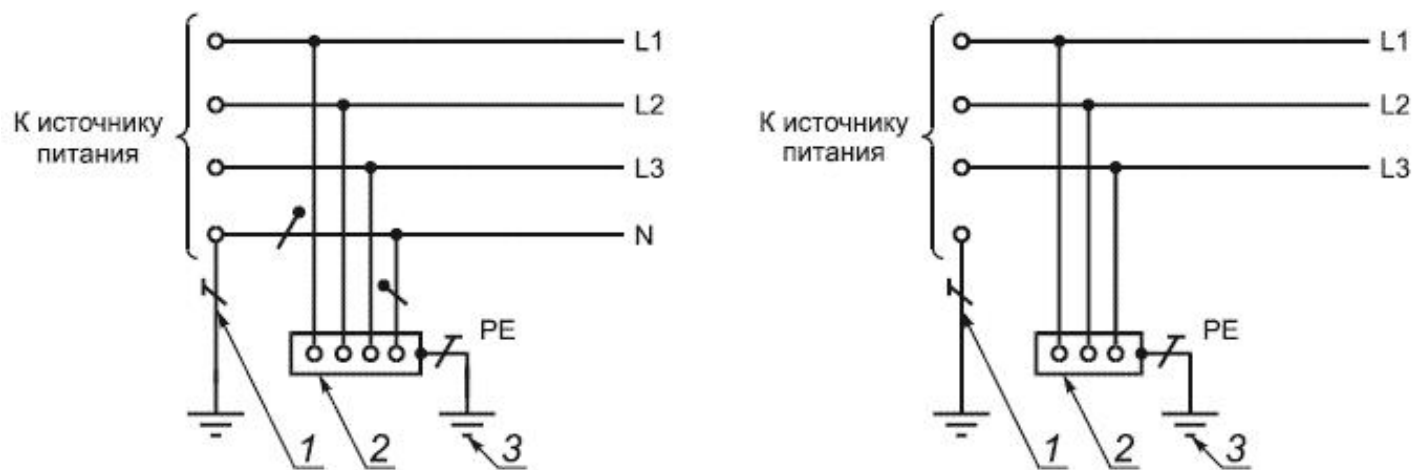
Рисунок Б.5 - Система TT переменного и постоянного тока
