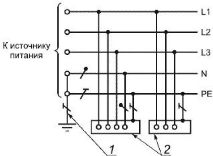
а) переменного тока
