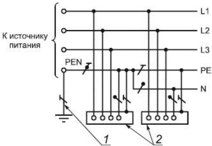
Рисунок Б.3 - Система TN-C-S переменного и постоянного тока
